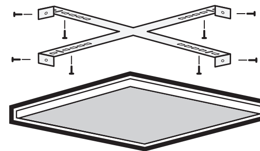
Рис. 1 Схема накладного монтажа светильника PPL SPEC
